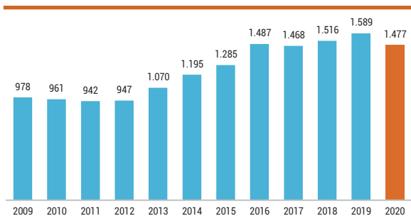
Bolivia: Producción Nacional de Gas Licuado de Petróleo (GLP), 2009 - 2020 (En toneladas métricas por día)
